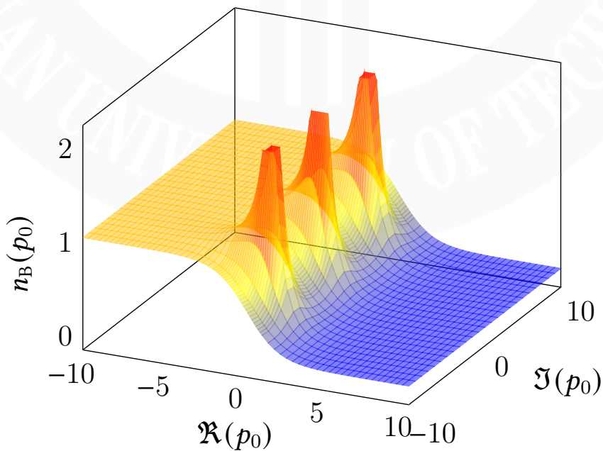
图 3-5 玻色爱因斯坦分布示意图
